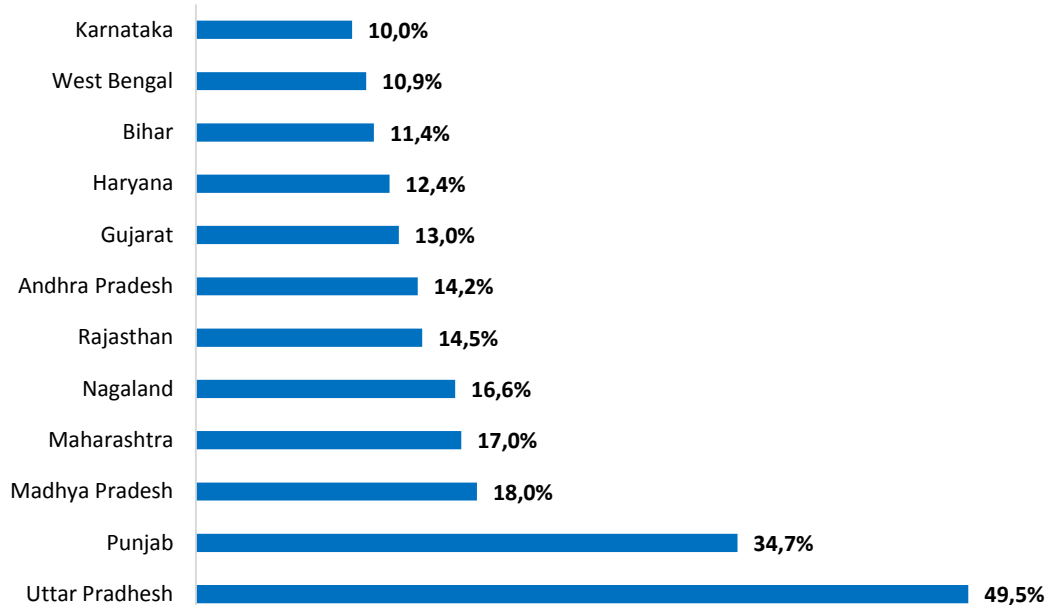
Abbildung 5.2: Regionaler Wasserverbrauch (in %)
