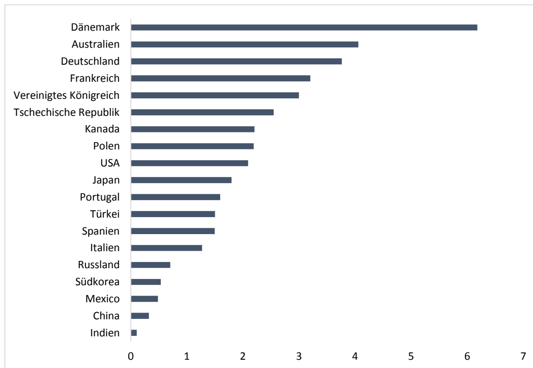
Abbildung 5.5: Tarife für Wasser und Abwasser für ausgewählte Länder im Jahr 2011 (in Euro/m³) Quelle: modifiziert nach Statista, 2018 [89]
