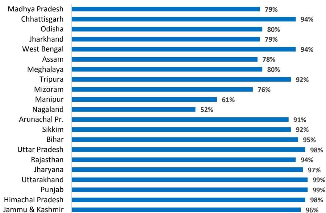
Abbildung 5.3: Wasserversorgungsgrad mit Trinkwasser nach Regionen (in %)
